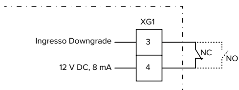
Fig. 18: Diagramma unifilare: collegamento di un contatto di commutazione esterno (impostazione di default: NO)
