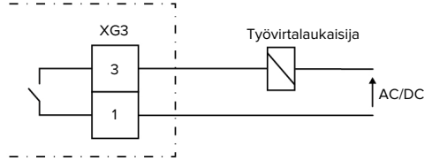
Kuva 12: Periaatekytkentäkaavio: ulkoisen työvirran laukaisijan liitäntä
