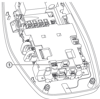
Ilustr. 15: Przyłączyć Ethernet
