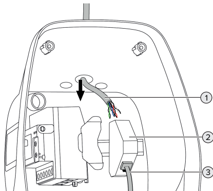
Fig. 16: Tilslutte netværkskablet (eksempel)
