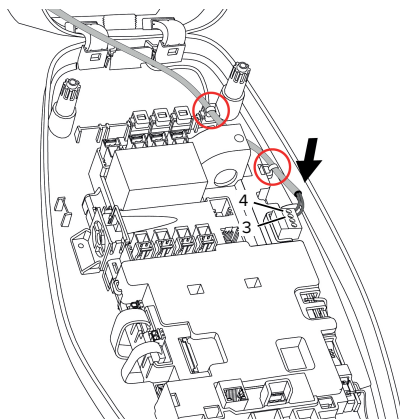
Fig. 17: Tilslutning downgrade-indgang
