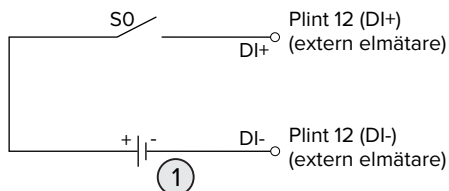
Fig. 19: Styrning via ett kopplingsrelä och ytterligare en spänningsförsörjning (vid leveranstillstånd)
