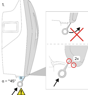
Fig. 4: Lossa frontkåpan – 1
