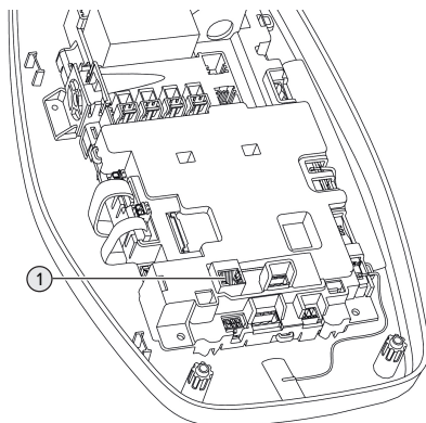
Kuva 15: Ethernet-liitäntä
