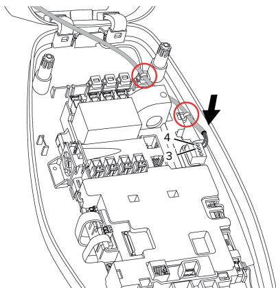
Fig. 17: Collegamento ingresso Downgrade
