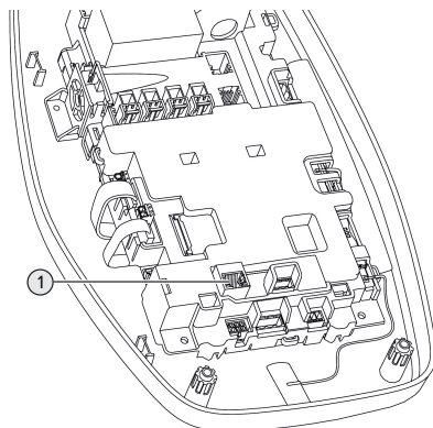
Fig. 15: Ethernet-anslutning
