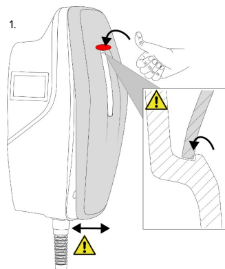
Afb. 22: Frontcover aanbrengen - 1
