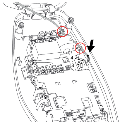
Abb. 17: Anschluss Downgrade-Eingang
