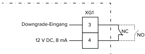
Abb. 18: Prinzipschaltbild: Anschluss eines externen Schaltkontakts (Standard-Einstellung: NO)
