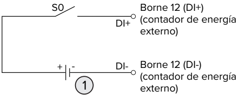
Fig. 19: Accionamiento mediante un relé acoplador y una alimentación de tensión adicional (en el estado de entrega)
