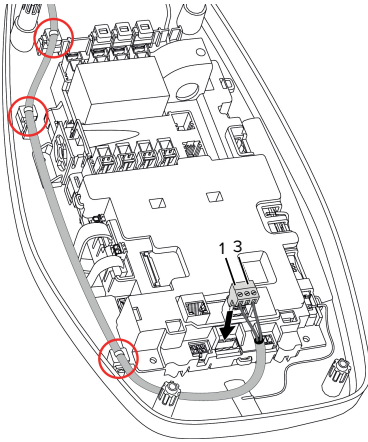
Kuva 11: Työvirtalaukaisijan liitäntä
