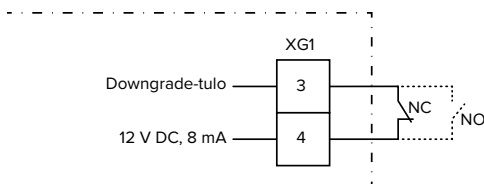
Kuva 18: PeriaatekytKentäkaavio: ulkoisen kytKentäkontaktin liitäntä (vakioasetus: NO)
