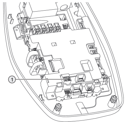
Abb. 15: Ethernet-Anschluss
