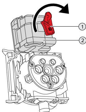
Fig. 26: Sblocco manuale della spina di ricarica
