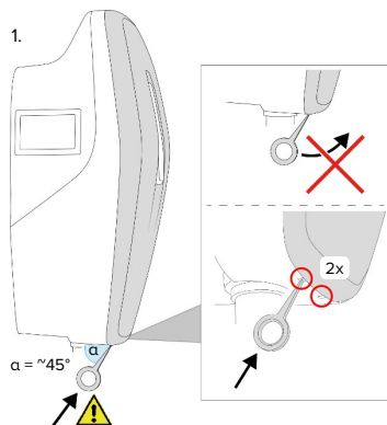
Ilustr. 4: Zdejmowanie pokrywy przedniej - 1
