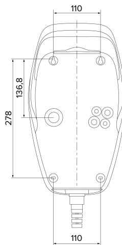
Fig. 7: Bormått [mm]
