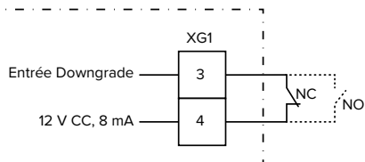
Fig. 18 : Schéma de principe : raccordement d'un contact électrique externe (réglage par défaut : NO)
