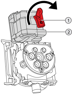
Abb. 26: Ladestecker manuell entriegeln
