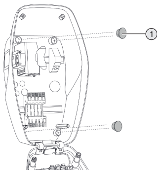
Afb. 9: Afsluitstoppen
