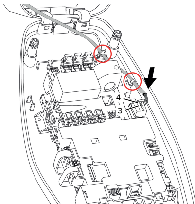
Kuva 17: Downgrade-tulon liitäntä
