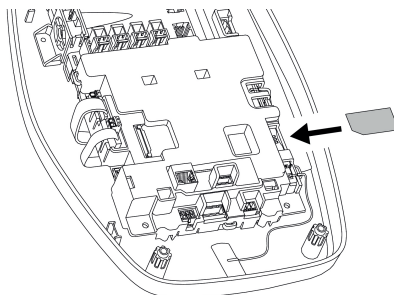
Fig. 13: Insertar la tarjeta SIM
