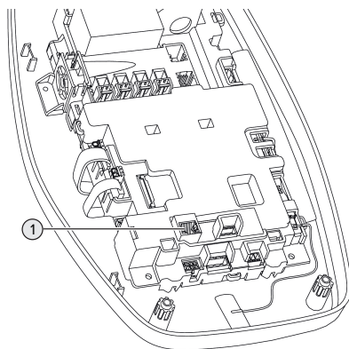
Fig. 15 : Prise Ethernet
