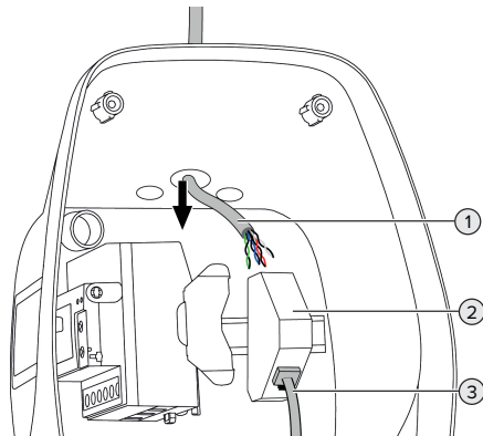
Afb. 16: Dataleiding aansluiten (voorbeeld)
