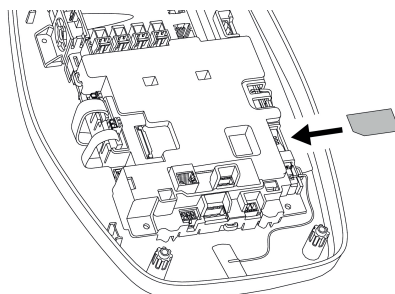
Fig. 13: Isætning af SIM-kort
