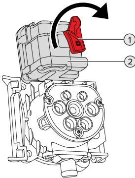
Afb. 26: Laadstekker handmatig ontgrendelen
