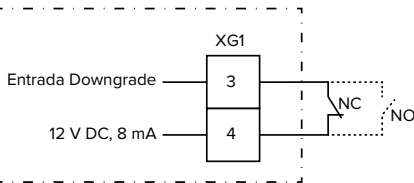
Fig. 18: Esquema de principio: Conexión de un contacto de conmutación externo (ajuste estándar: NC)
