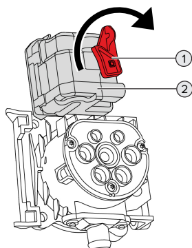
Fig. 26 : Déverrouillage manuel de la fiche de charge
