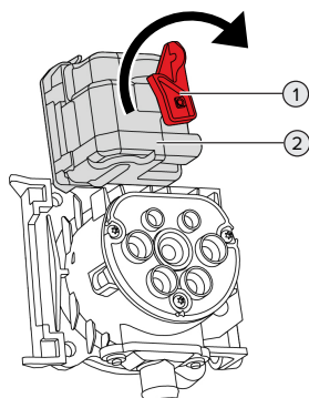
Fig. 26: Frigör laddkontakten manuellt
