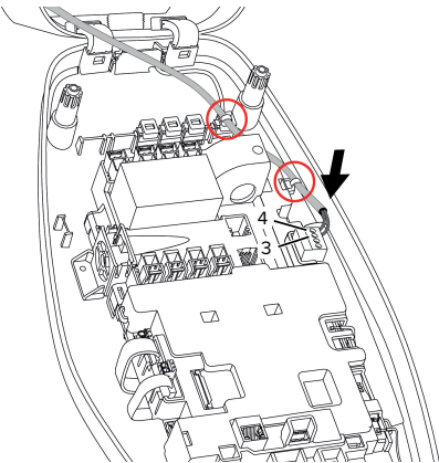
Fig. 17: Conexión entrada Downgrade
