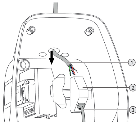
Fig. 16 : Branchement de la ligne de données (exemple)
