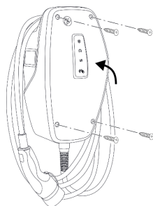
Afb. 20: Product sluiten
