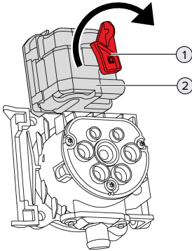
Fig. 26: Desbloquear el conector de carga manualmente
