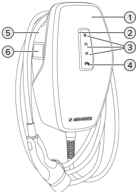
Kuva 2: Ulkonäkymä (esimerkki)
