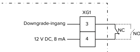
Afb. 18: Principeschema: aansluiting van een extern schakelcontact (standaardinstelling: NO)
