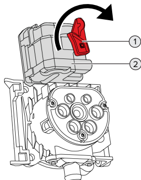
Ilustr. 26: Odblokowanie ręczne wtyczki ładowania
