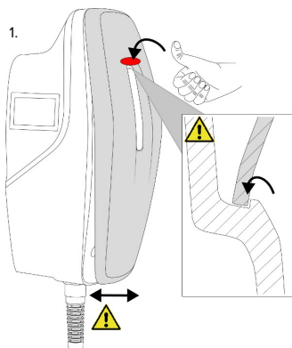
Ilustr. 22: Zakładanie pokrywy przedniej - 1
