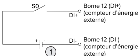
Fig. 19 : Activation par le biais d'un relais de couplage et d'une alimentation électrique supplémentaire (à l'état à la livraison)
