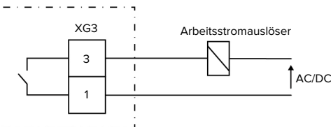
Abb. 12: Prinzipschaltbild: Anschluss eines externen Arbeitsstromauslösers
