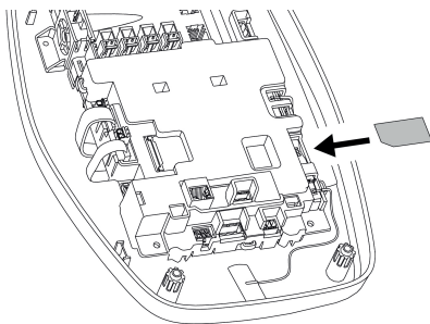
Fig. 13 : Insertion de la carte SIM
