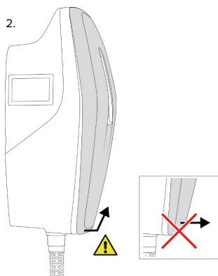
Fig. 5: Lossa frontkåpan – 2
