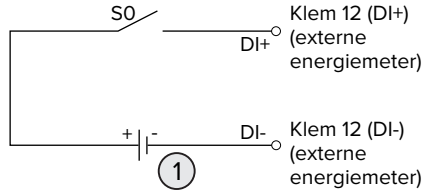
Afb. 19: Aansturing via een koppelrelais en een extra stroomvoorziening (in de uitleveringstoestand)
