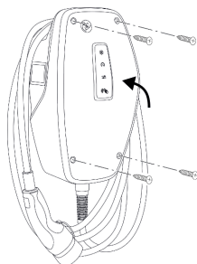
Fig. 20: Stäng produkten
