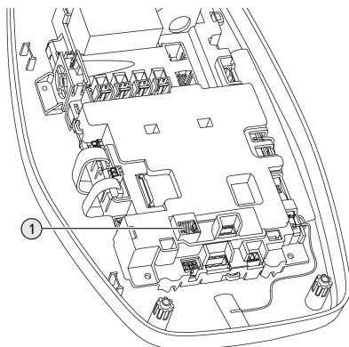
Fig. 15: Ethernet port
