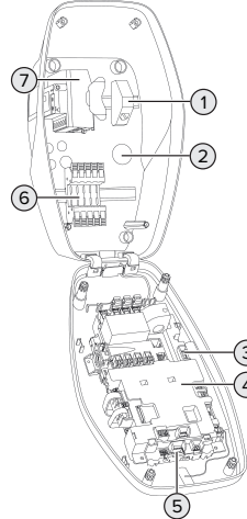
Kuva 3: Sisänäkymä (esimerkki)
