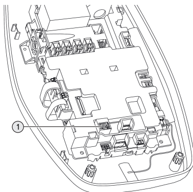
Afb. 15: Ethernet aansluiting
