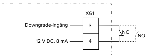
Fig. 18: Principkopplingsschema: anslutning av en extern brytarkontakt (standardinställning: NO)
