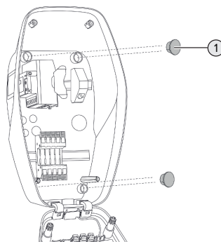
Fig. 9: Tappo
