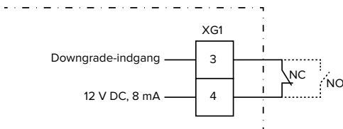
Fig. 18: Principskema: tilslutning af en ekstern omskifterkontakt (standardindstilling: NO)
