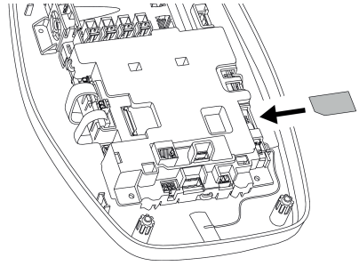
Abb. 13: SIM-Karte einsetzen
