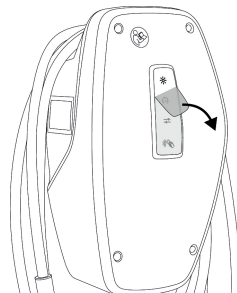
Fig. 21 : Retirer le film de protection
