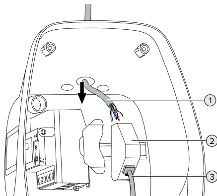
Ilustr. 16: Podłączenie przewodu danych (przykład)
