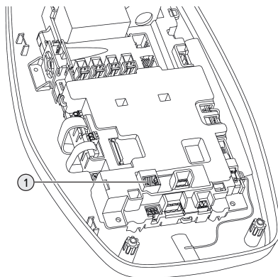
Fig. 15: Ethernet-tilslutning
