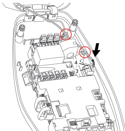
Fig. 17: Anslutning av downgrade-ingång
