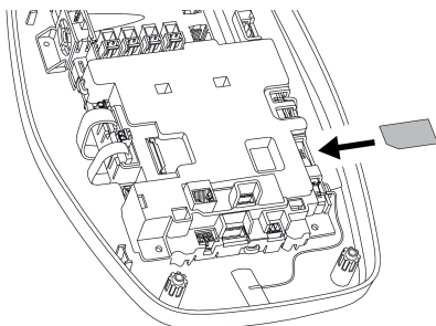
Fig. 13: Inserimento della scheda SIM
