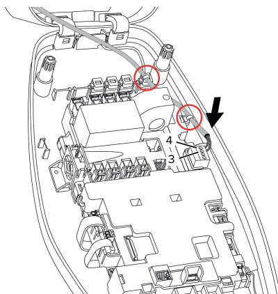
Afb. 17: Aansluiting downgrade-ingang
