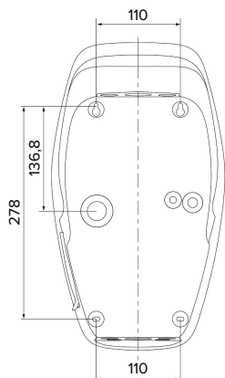
Fig. 8: Borrmått [mm]
