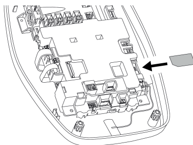
Kuva 13: SIM-kortin asettaminen
