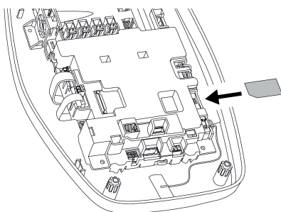
Fig. 13: Sätta i SIM-kort
