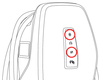
Fig. 14: Activar punto de acceso
