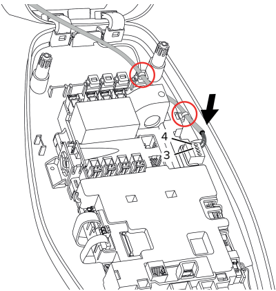
Ilustr. 17: Przyłącze wejścia downgrade
