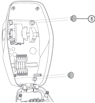
Fig. 9: Lukkepropper
