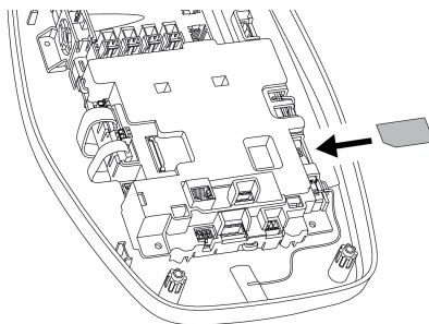
Ilustr. 13: Wkładanie karty SIM
