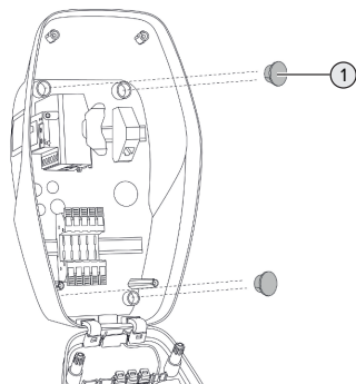
Fig. 9: Täcklock
