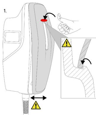
Fig. 22 : Monter le cache frontal - 1
