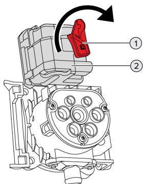
Fig. 26: Løsne ladestikket manuelt
