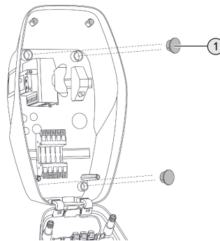
Abb. 9: Verschlussstopfen
