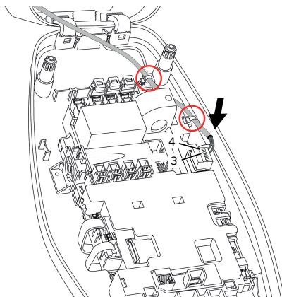
Fig. 17 : Raccordement de l'entrée Downgrade
