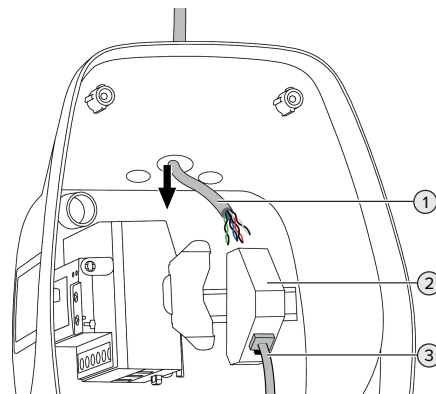
Fig. 16: Collegamento della linea di trasmissione dati (esempio)
