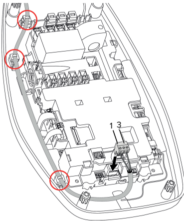
Abb. 11: Anschluss Arbeitsstromauslöser
