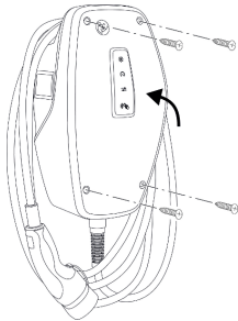
Abb. 20: Produkt schließen
