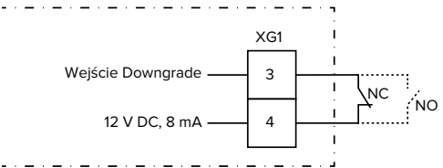
Ilustr. 18: Schemat obwodu: podłączenie zewnętrznego styku przełączającego (ustawienie standardowe: NO)
