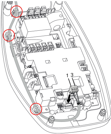
Fig. 11: Collegamento sganciatore di apertura
