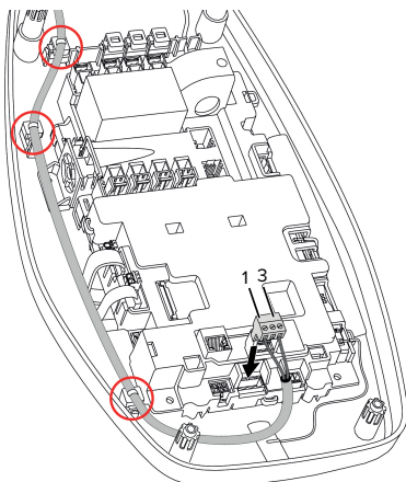
Fig. 11: Tilkobling arbejdsstrømsudløser
