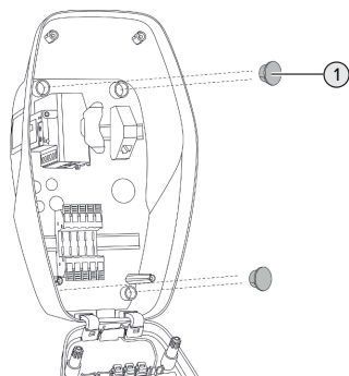
Ilustr. 9: Zatyczka
