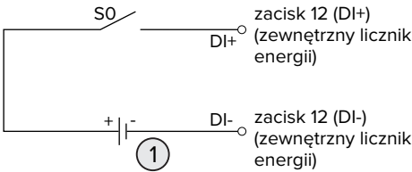
Ilustr. 19: Sterowanie przez przełącznik parujący i dodatkowe zasilanie napięciowe (w stanie dostawy)
