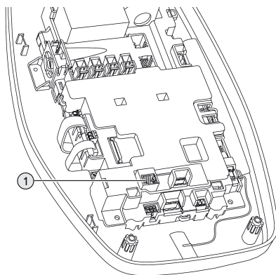
Fig. 15: Conexión Ethernet
