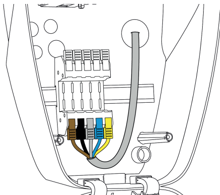
Ilustr. 10: Przyłącze zasilania napięciowego (przekład)
