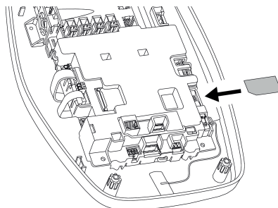
Afb. 13: SIM-kaart plaatsen
