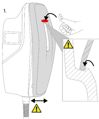
Fig. 22: Montaggio della cover anteriore - 1
