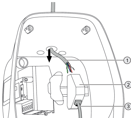
Fig. 16: Anslut dataledning (exempel)
