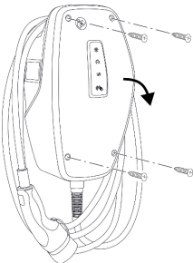
Fig. 6 : Ouverture du produit
