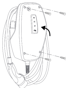
Fig. 20: Lukke produktet
